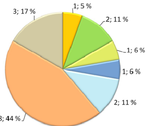
Kuva 2. Järjestelmätyypit (n=18)
